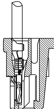
插线状态
